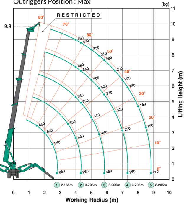
850kg Searcher Hook (Offset Position : SH2) Outriggers Position : Max
